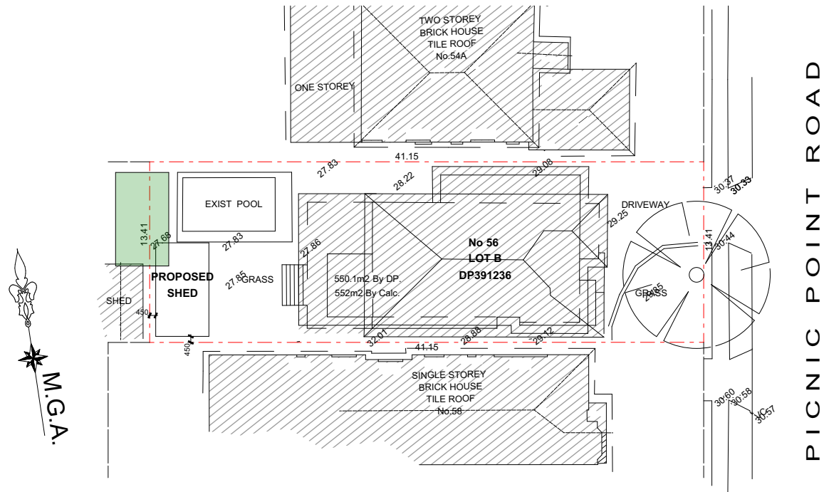
Site Plan 1:400
